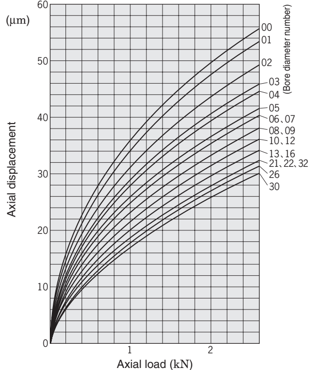
(4) 7200C, 7200CPA series (contact angle : 15°)
