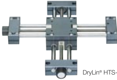
DryLin® HTS
