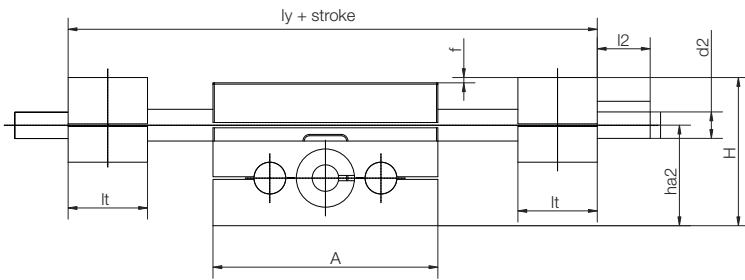
DryLin® HTS-PL
