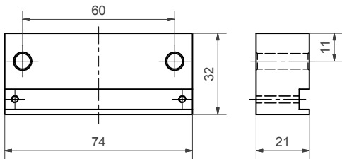
STY-104001
