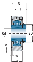
UKC200H UKC300H
