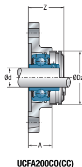
UCFA200C(CC)
