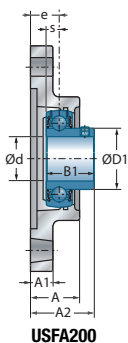
USFA200
