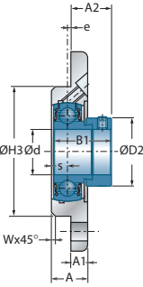
ESFCE200
